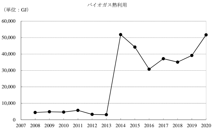
図 37 バイオガス熱利用量の経年変化
